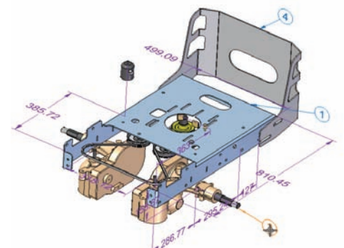
Abbildung 10. Konstrukteure können jetzt Positionsnummern in der Baugruppe vergeben, die bei der Zeichnungserstellung übernommen werden können.
