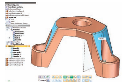
Abbildung 4. Die Konstrukteure können zur schnelleren Modellierung selektiv die Features, die die Basisform definieren, in den synchronen Bereich verschieben, andere Features dabei aber im sequentiellen Modus belassen.
